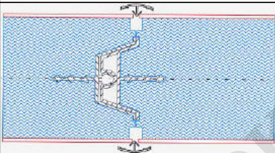
Interlock - Schnappverbindung u. PVC-Deckprofilen
