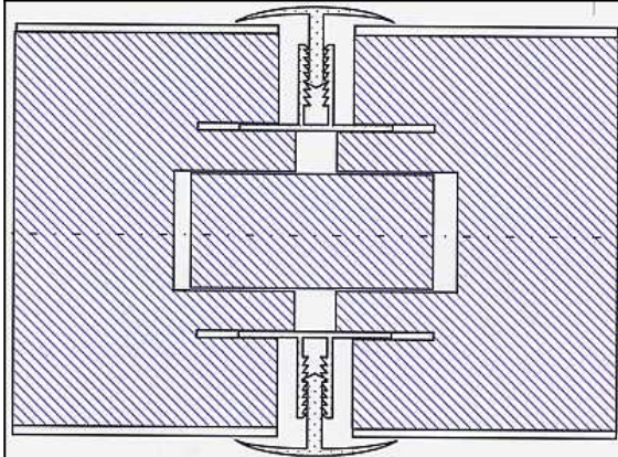
Verbindung mittels Styroporfeder u. PVC-Deckprofilen (H20)
